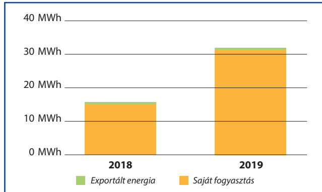
Az Egészségház megtermelt villamos energiája az inverternél mérve 2019. augusztusig
