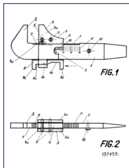
Kiss A. Ferdinánd egyik franciakulcsának szabadalmi terve
