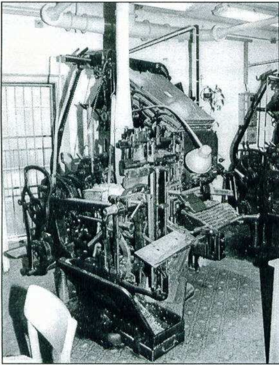
Sorszedőgép, amellyel a kéziratokból ólomsorok lettek.
