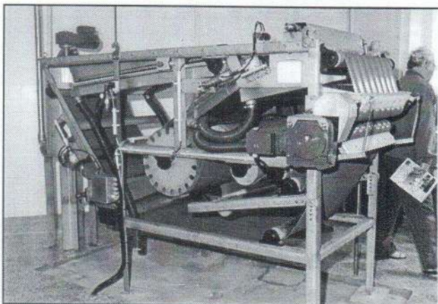
A szalagszűrőprés
